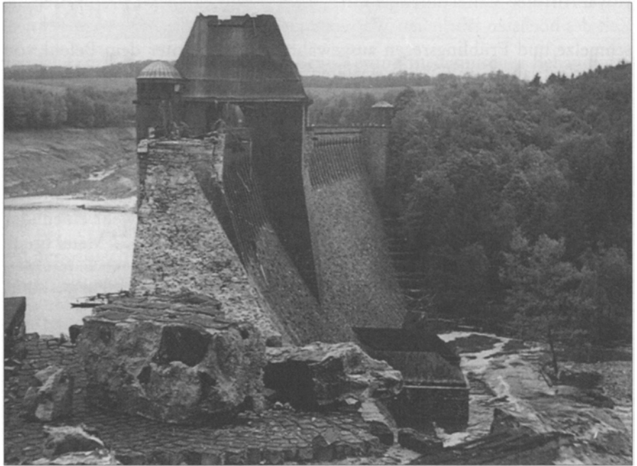
Die Staumauer der Möhnetalsperre nach dem britischen Angriff vom 17. Mai 1943. Aus: Chronik des Zweiten Weltkriegs , Chronik, Gütersloh 1999
